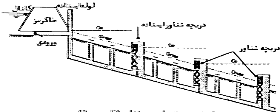
(iii) سیستم نیمه بسته یا دریچه شناور تفلی
