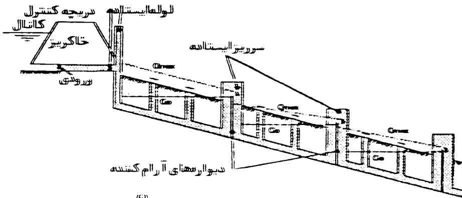
(ii) سیستم باز یا سرریز ایستاده - تفلی
